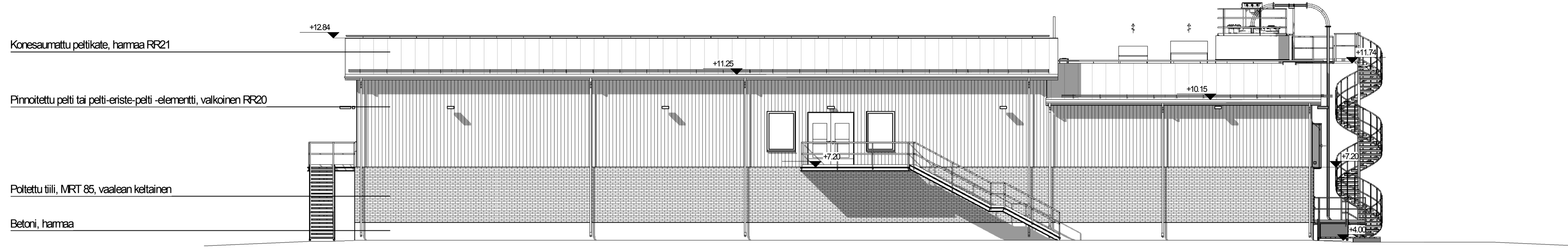
Julkisivu itään
