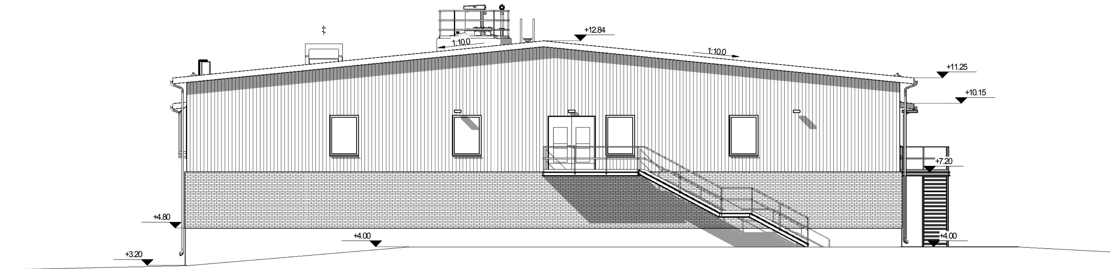
Julkisivu etelään
