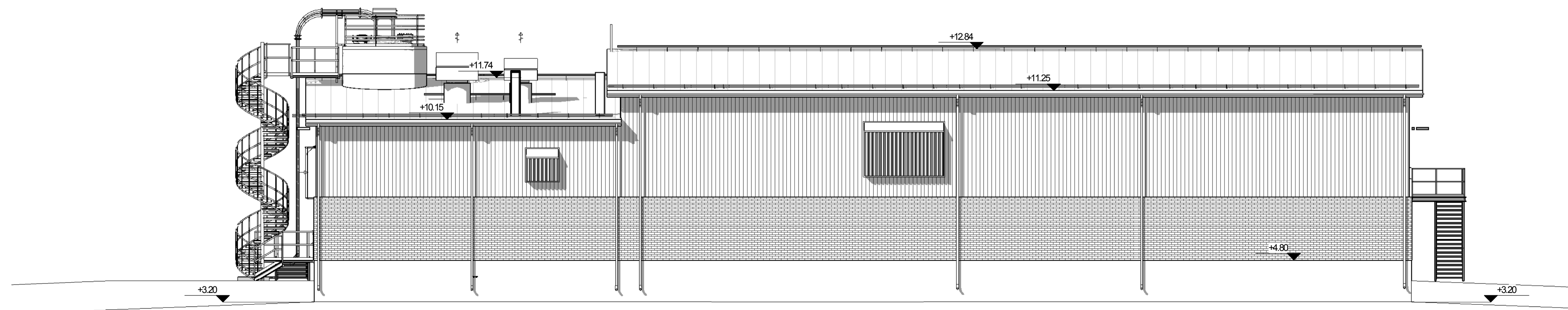
Julkisivu länteen
