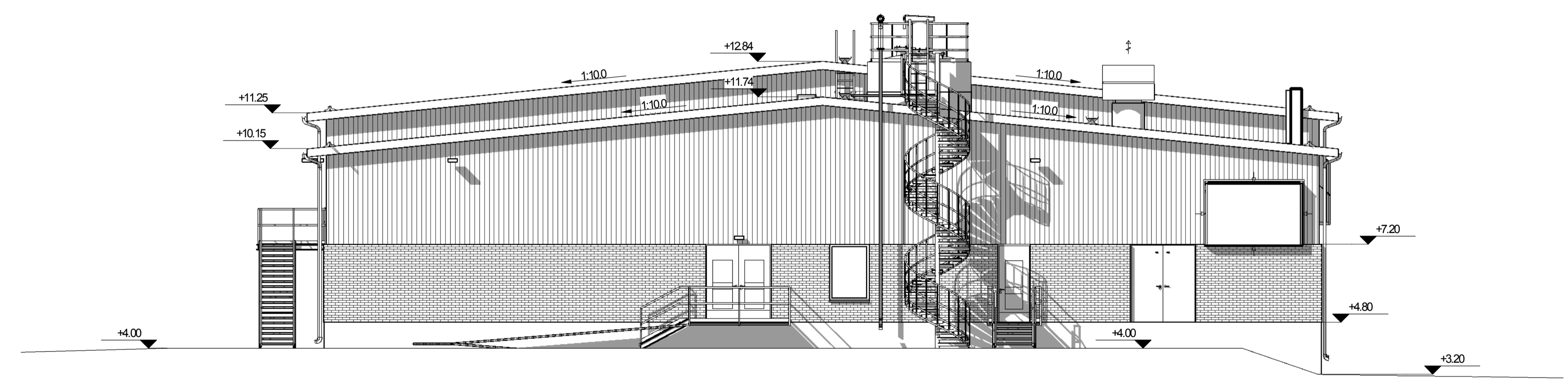
Julkisivu pohjoiseen
